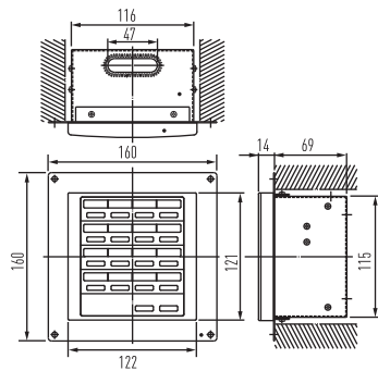
ПУЛЬТ УПРАВЛЕНИЯ ВКЛ./ ВЫКЛ. (CZ-ANC2)
