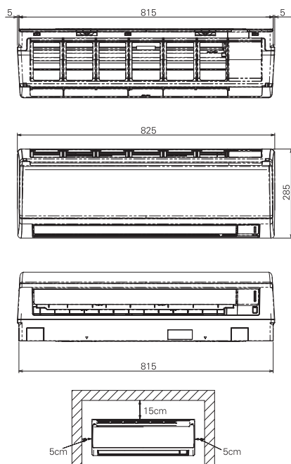
Передний вид
