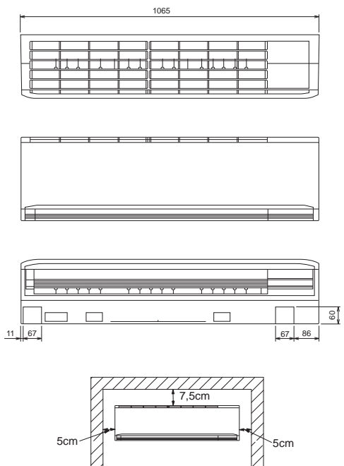
Передний вид
