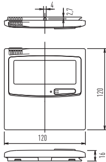
СИСТЕМНЫЙ ПУЛЬТ УПРАВЛЕНИЯ (CZ-64ESMC2)
