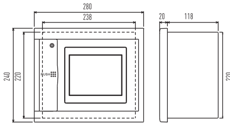
ИНТЕЛЛЕКТУАЛЬНЫЙ КОНТРОЛЛЕР (CZ-256ESMC2)
